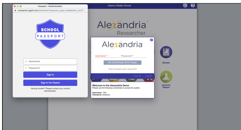
GG4L Login
